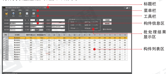
图 3-3 软件主界面
