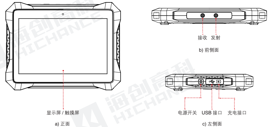
图 2.1 HC-U91 混凝土超声波检测仪主机外观示意图
