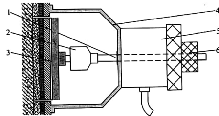
图 4.0.4 粘结强度检测仪安装示意 1—拉力杆；2—万向接头；3—标准块；4—支架； 5—穿心式千斤顶；6—拉力杆螺母
