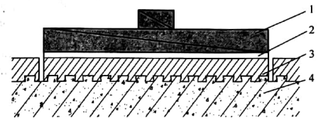
图 4.0.3-3 预制构件饰面砖试样胶粘标准块示意 1—标准块；2—胶粘剂；3—饰面砖；4—混凝土层
