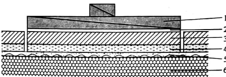
图 4.0.3-2 基体带加强或保温现场粘贴饰面砖试样胶粘标准块示意 1—标准块；2—胶粘剂；3—饰面砖；4—粘结层； 5—加强抹面层；6—保温层或低强度基体
