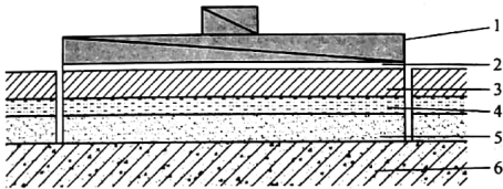
图 4.0.3-1 基体不带加强或保温现场粘贴饰面砖试样胶粘标准块示意 1—标准块；2—胶粘剂；3—饰面砖； 4—粘结层；5—找平层；6—基体
